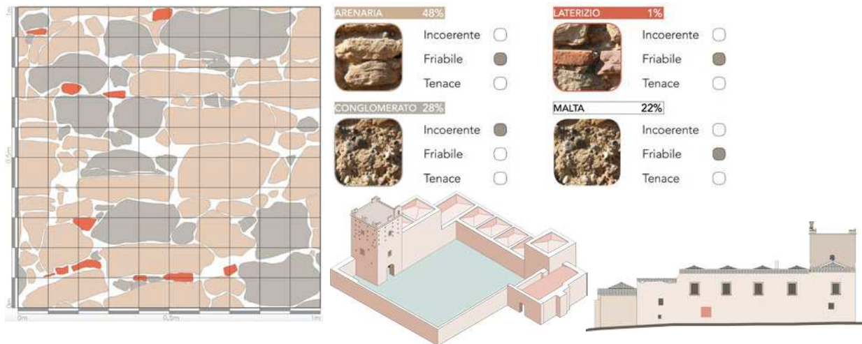
Figura 4: Analisi del paramento murario; assonometria e prospetto del quarto impianto.
