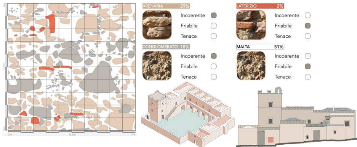
Figura 5: Analisi del paramento murario; assonometria e prospetto del quinto impianto.
