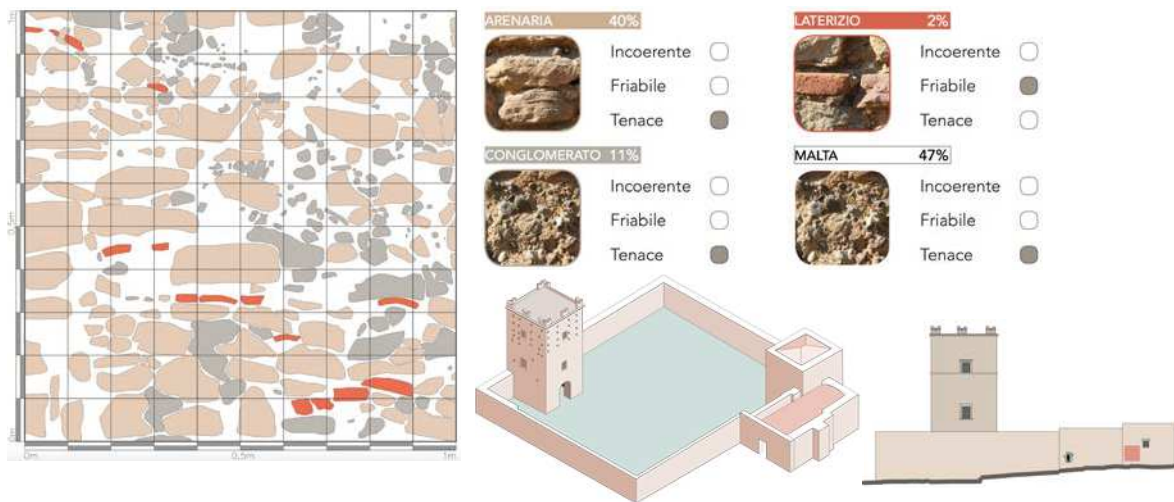
Figura 2: Analisi del paramento murario; assonometria e prospetto del secondo impianto.
