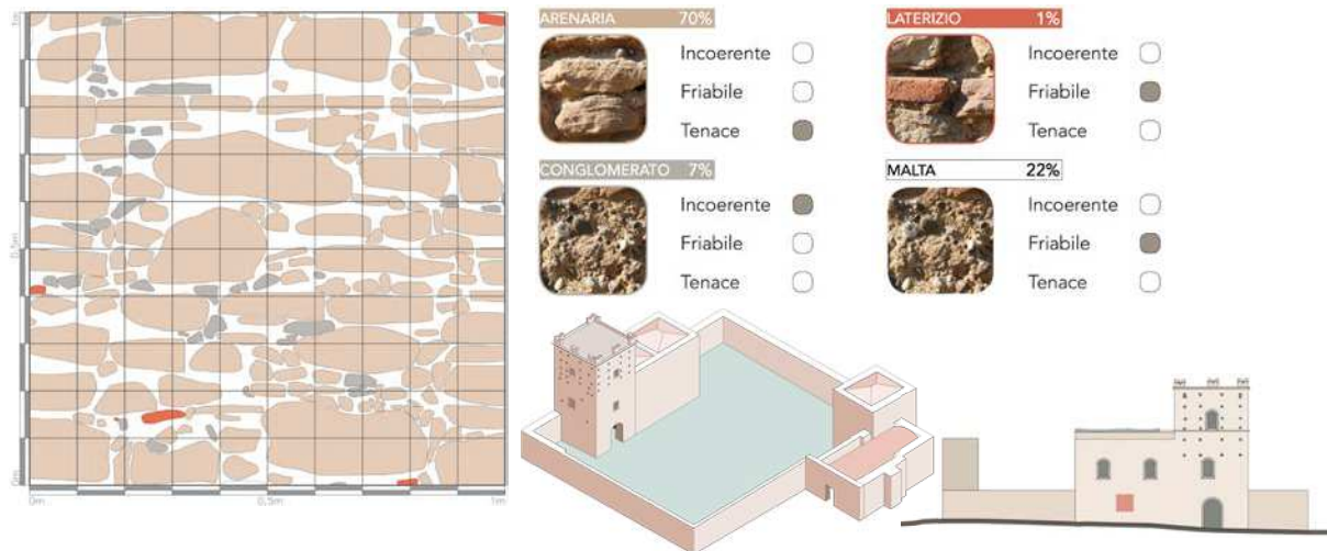
Figura 3: Analisi del paramento murario; assonometria e prospetto del terzo impianto.
