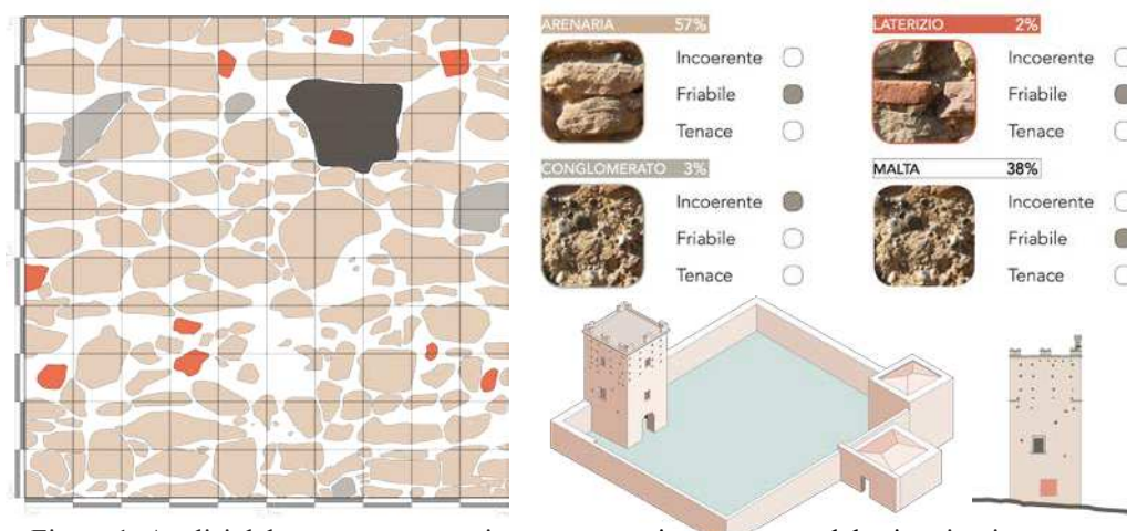
Figura 1: Analisi del paramento murario; assonometria e prospetto del primo impianto.
