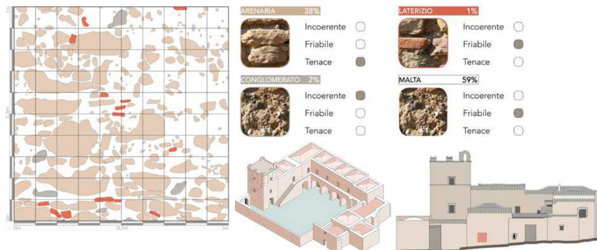
Figura 6: Analisi del paramento murario; assonometria e prospetto del sesto impianto.
