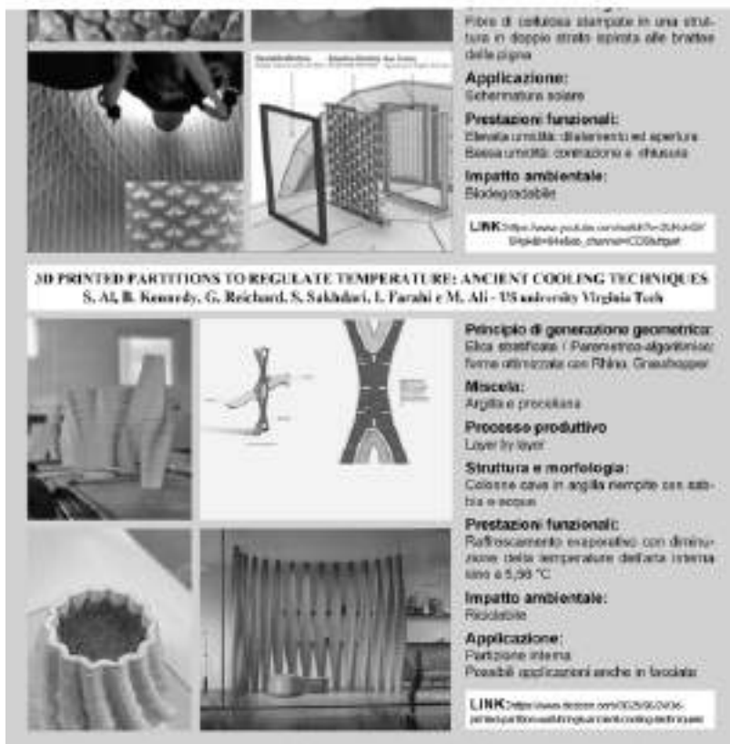
Figura 5. Esempi di componenti per schermature solari e partizione evaporative stampate in 3D [fonte: Elaborazione degli autori].
