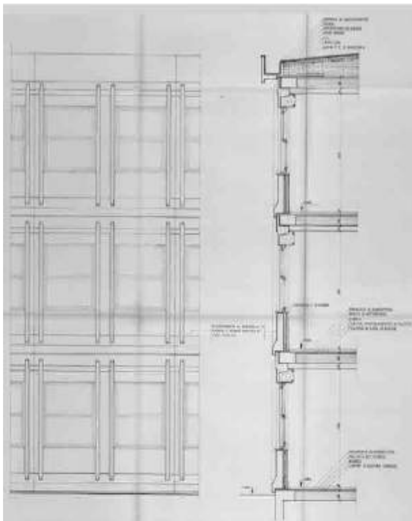
Figura 3. Scuola media a Fabriano: particolare costruttivo dei pannelli di facciata. [Fonte: ASTO-Borini, f. 3479].
