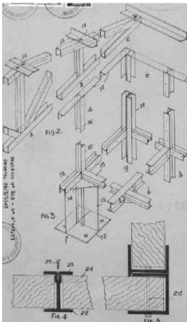
Figura 5. Dettagli nodi tipo della struttura e connessioni tra montanti e pannelli. [Fonte: ACS-UIBM, brevetto n. 412259 del 1946].
