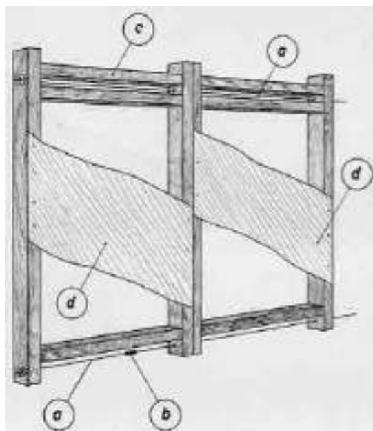
Figura 3. Brevetto Legnami Pasotti n. 353302 del 1937. [Fonte: ACS-UIBM].
