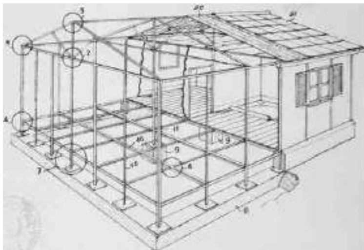
Figura 4. Schema costruttivo casa prefabbricata smontabile L'Invulnerabile, brevetto "Sistema per la costruzione rapida di case prefabbricate" [Fonte: ACS-UIBM, brevetto n. 412259 del 1946].
