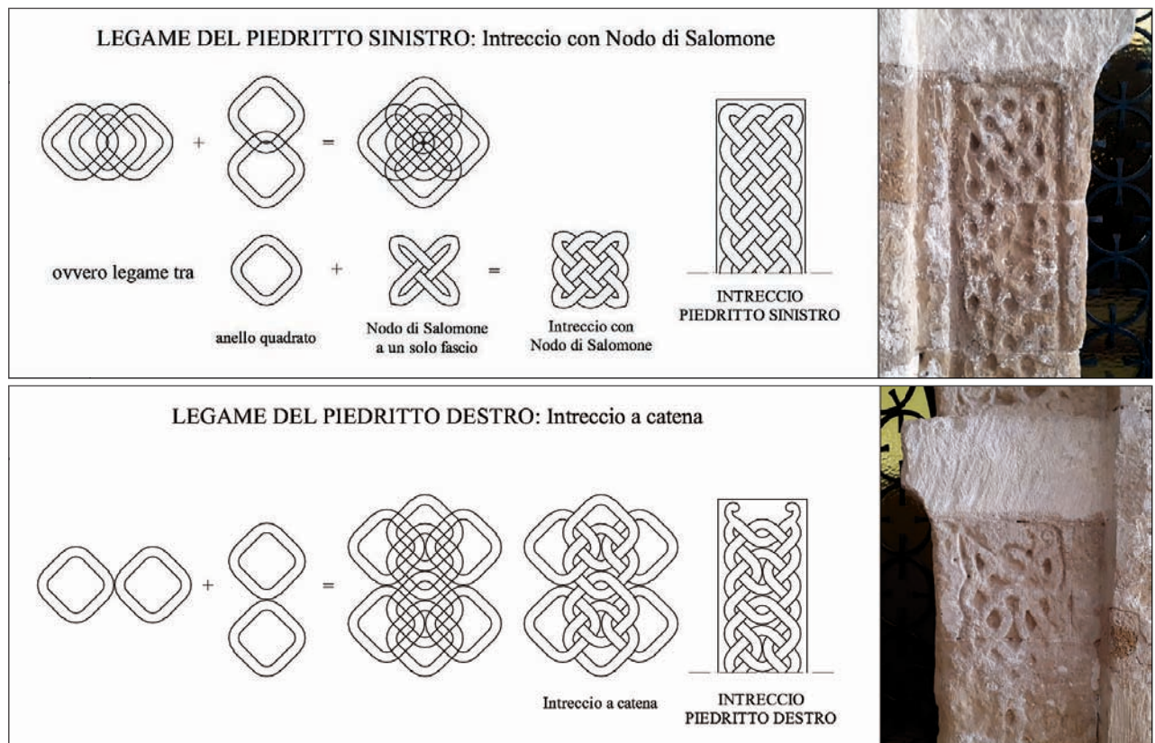
Fig. 13 e 14 - Piedritti
