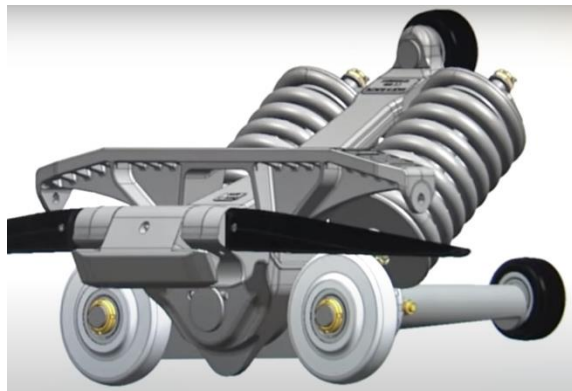
Figura 6: Morsa automatica per agganciamento temporaneo dei veicoli alla fune
